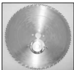
Lame seule Ø650 - 80 dents - épaisseur 4 mm réf. 35.600.680
